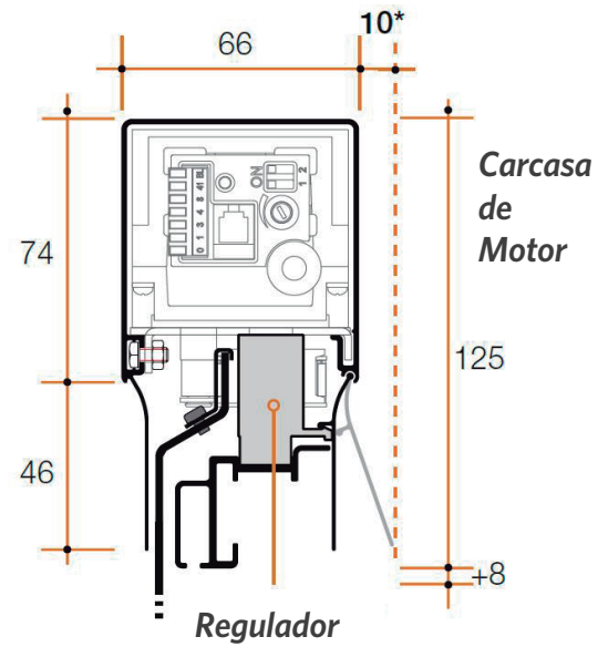
SECCIÓN VERTICAL
